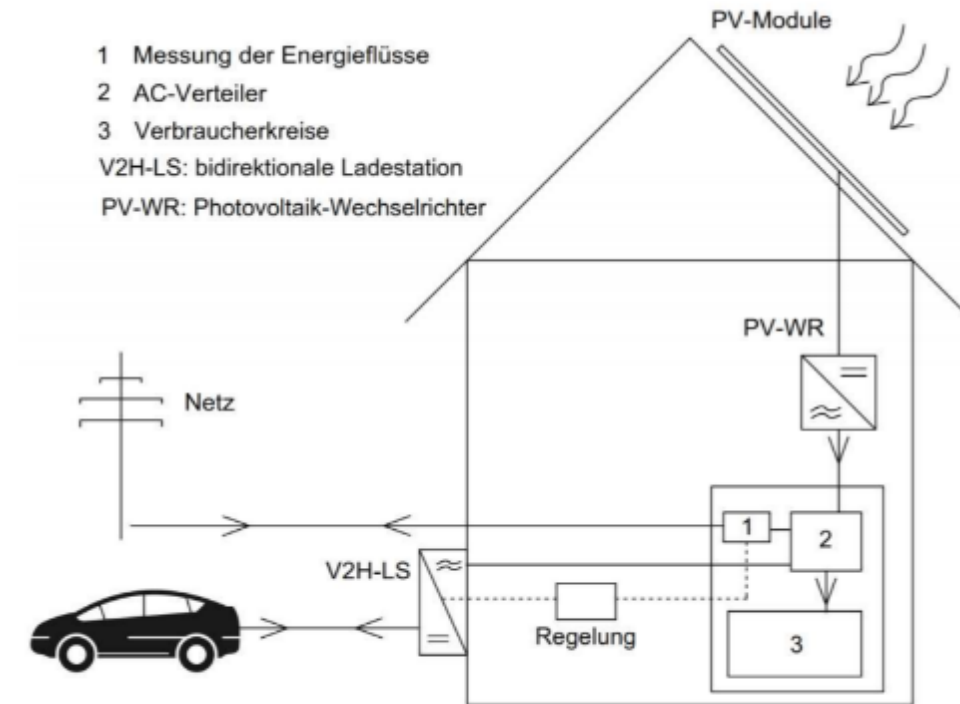
Abbildung 1: Komponenten eines Vehicle-to-Home Systems (eigene Darstellung)
